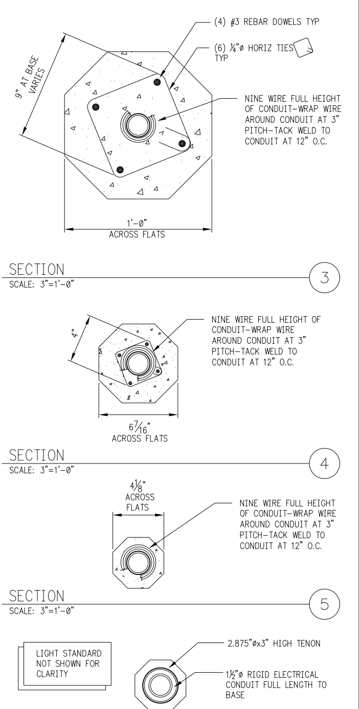
SECTION SCALE: 3"=1'-0"
