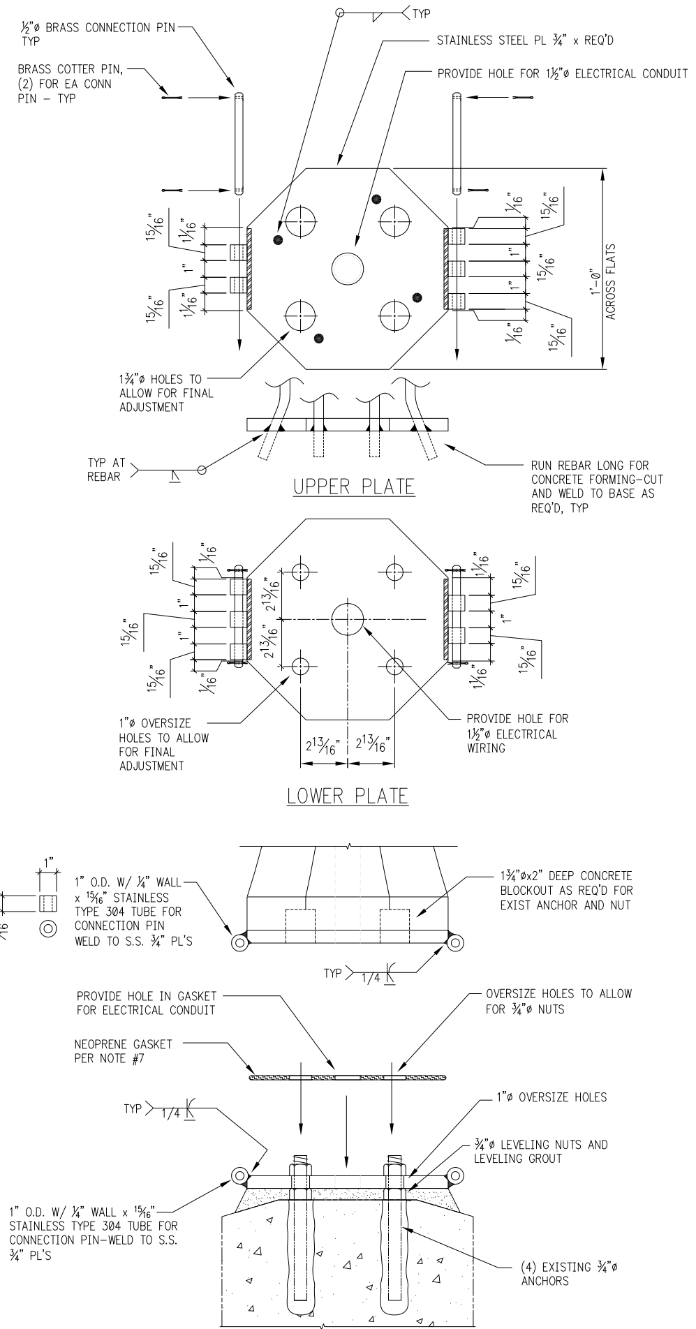
SECTION SCALE: 3"=1'-0"
