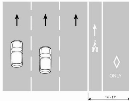
Optimal
